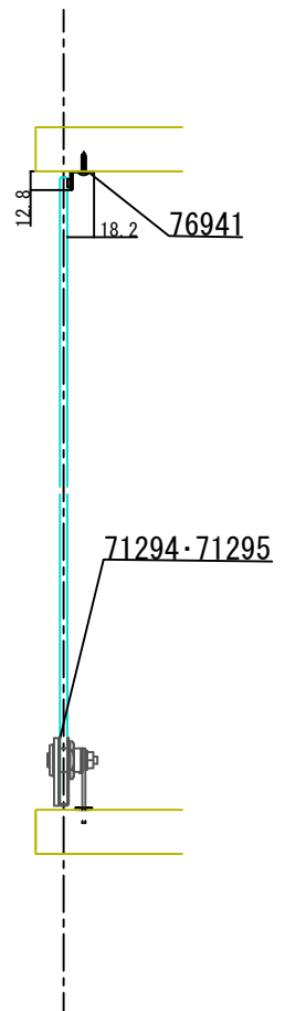
B-B断面図
