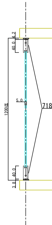
A-A断面図
