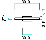
正面図
