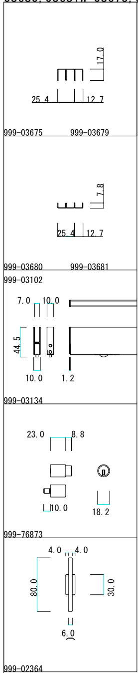
正面図
