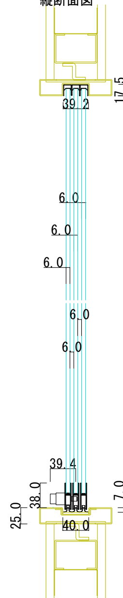
縦断面図
