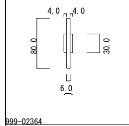
正面图
