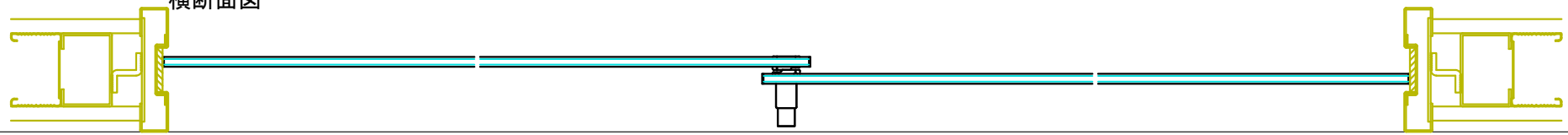
横断面図
