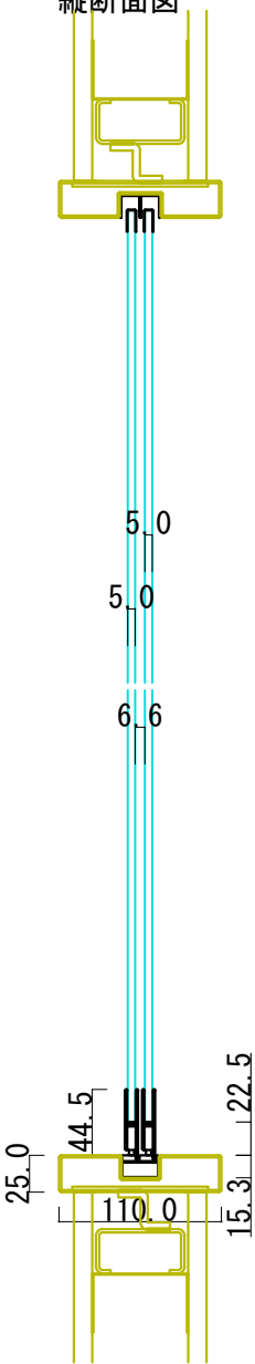
縦断面図
