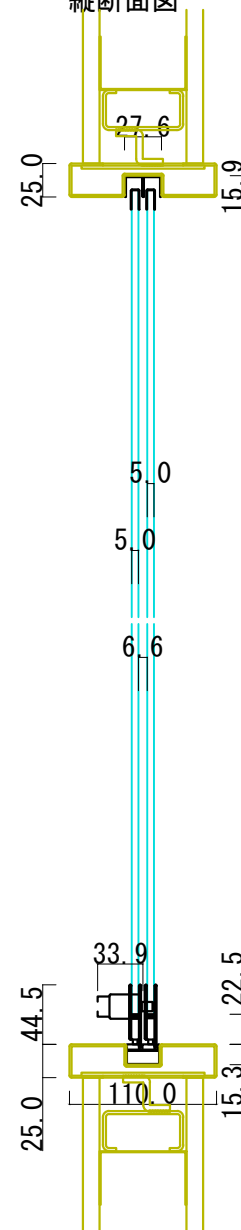
縦断面図
