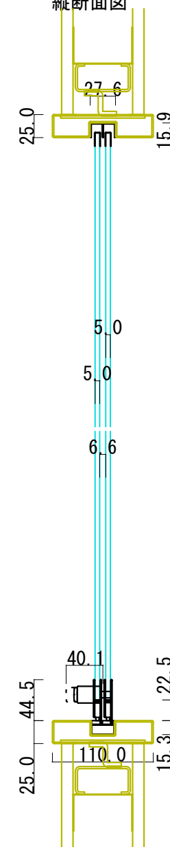
縦断面図
