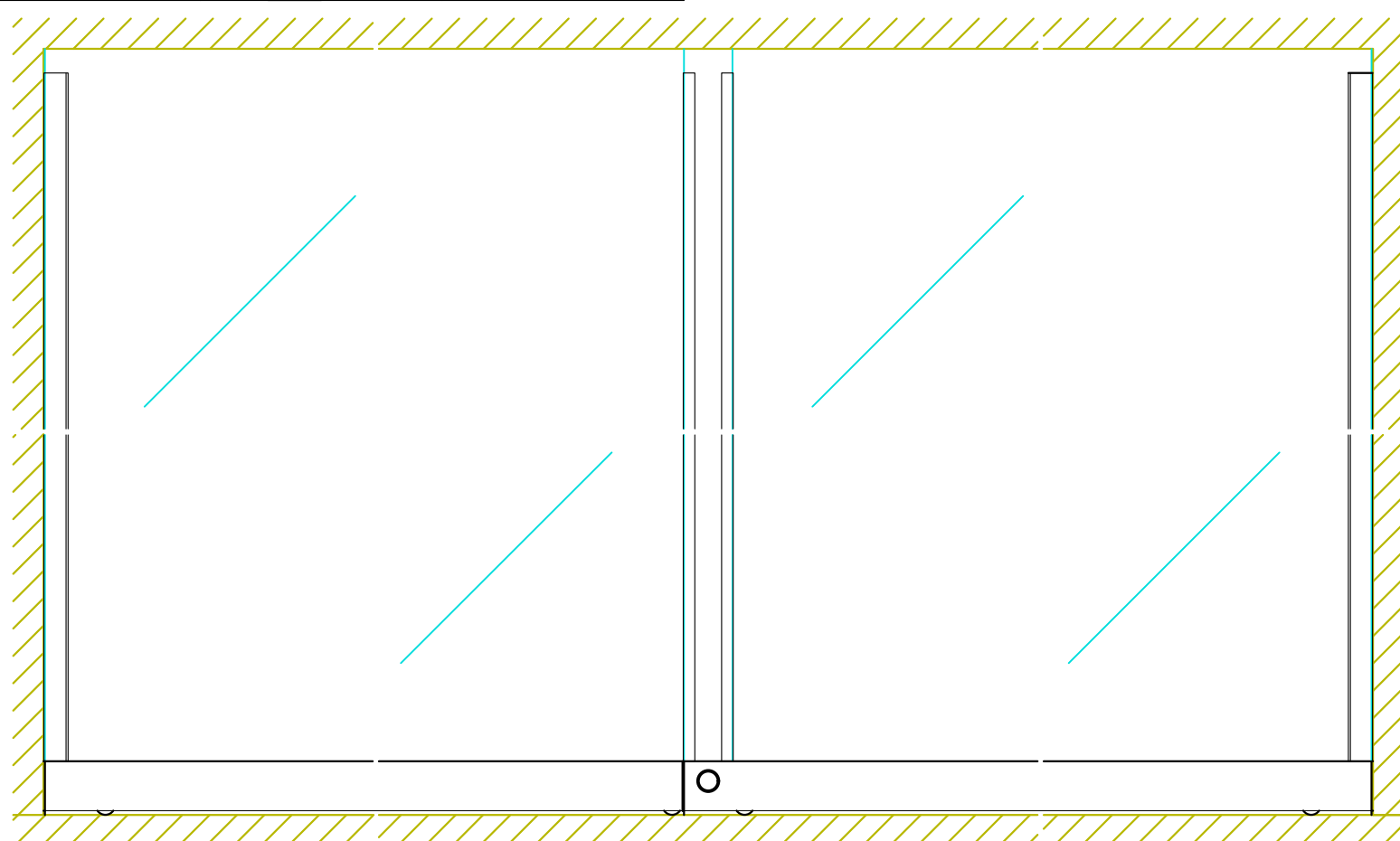
正面図
