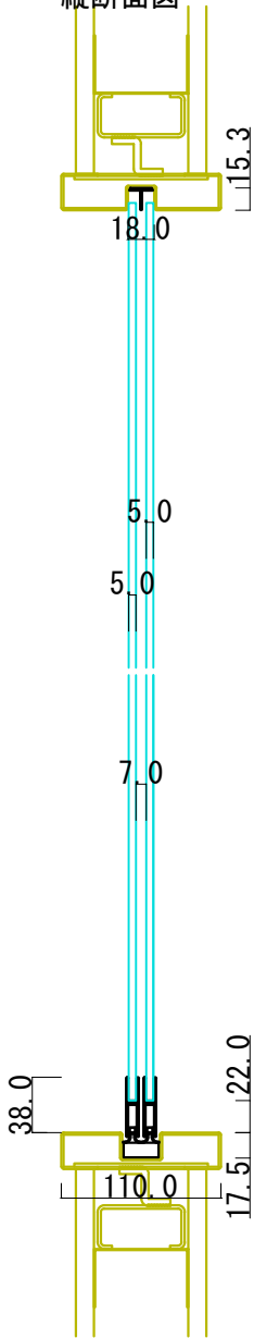
縦断面図
