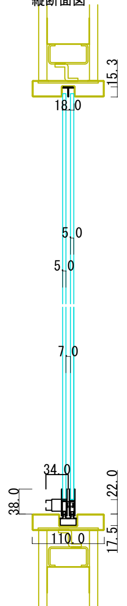
縦断面図
