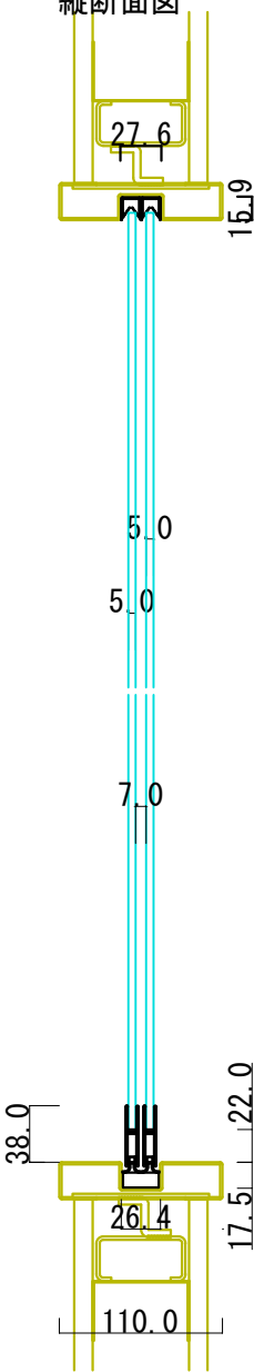
縦断面図
