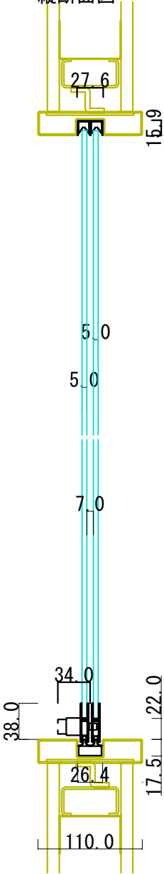
縦断面図
