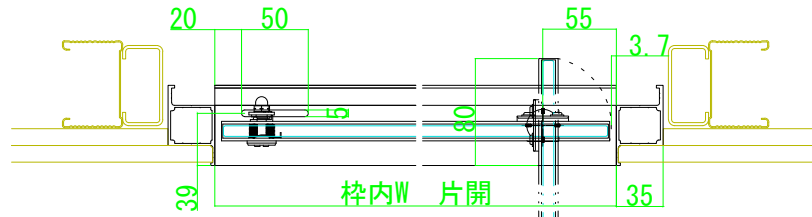
D-D断面図
