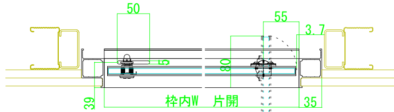
D-D断面図
