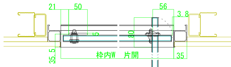
D-D断面図
