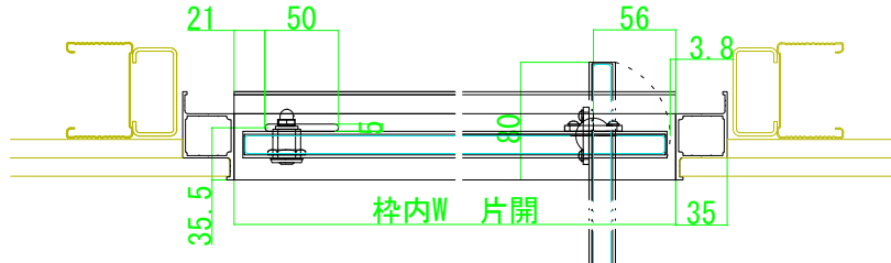
D-D断面図
