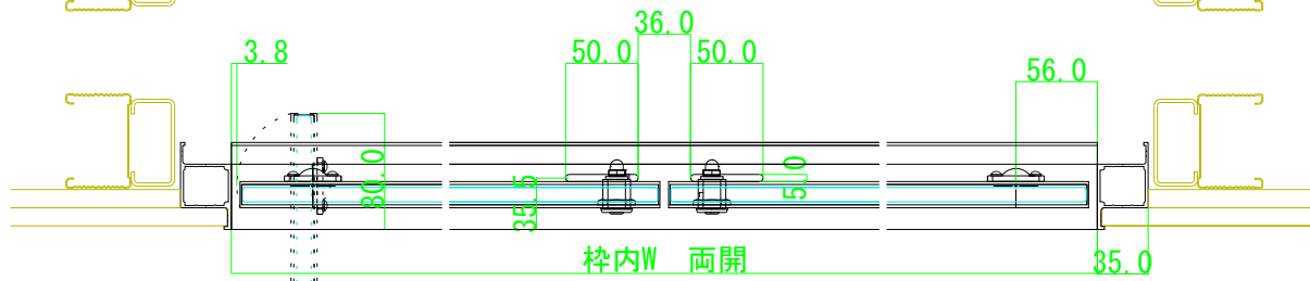
D-D断面図
