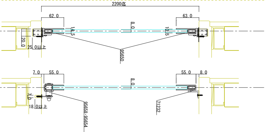
A-A断面図
