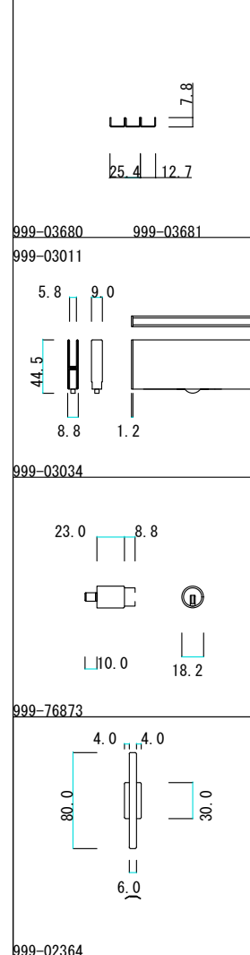
正面図
