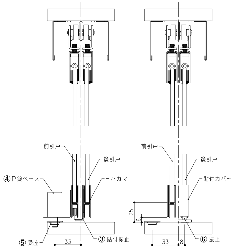
図1.断面：錠前側
