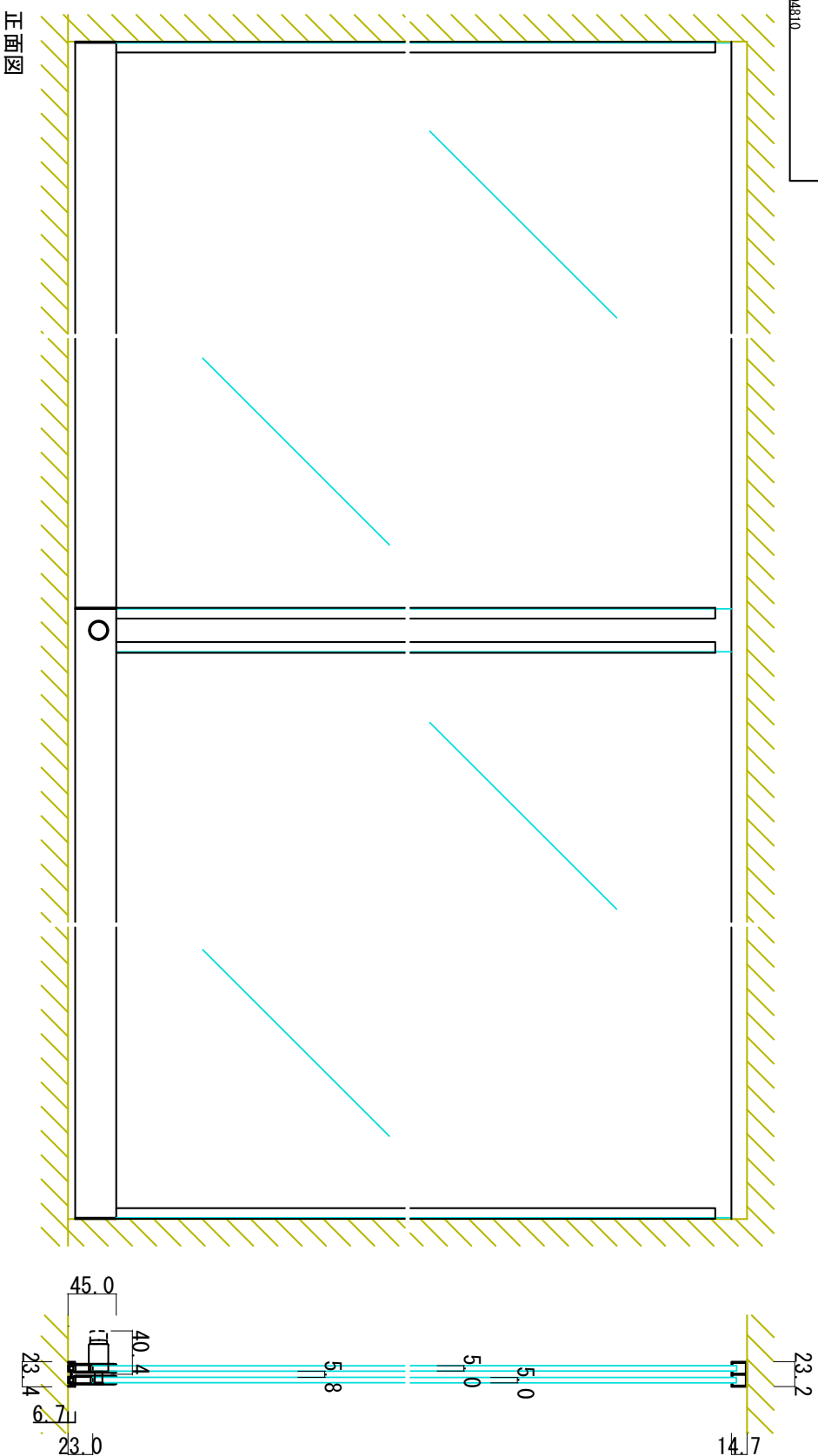
横断面図
